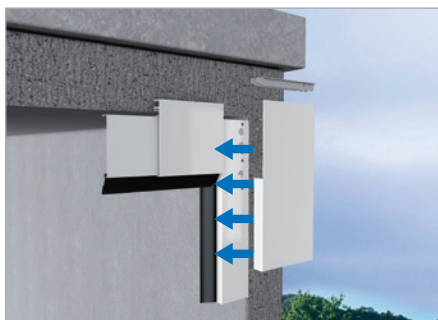
Universal-Blendenlösung, Außenansicht
